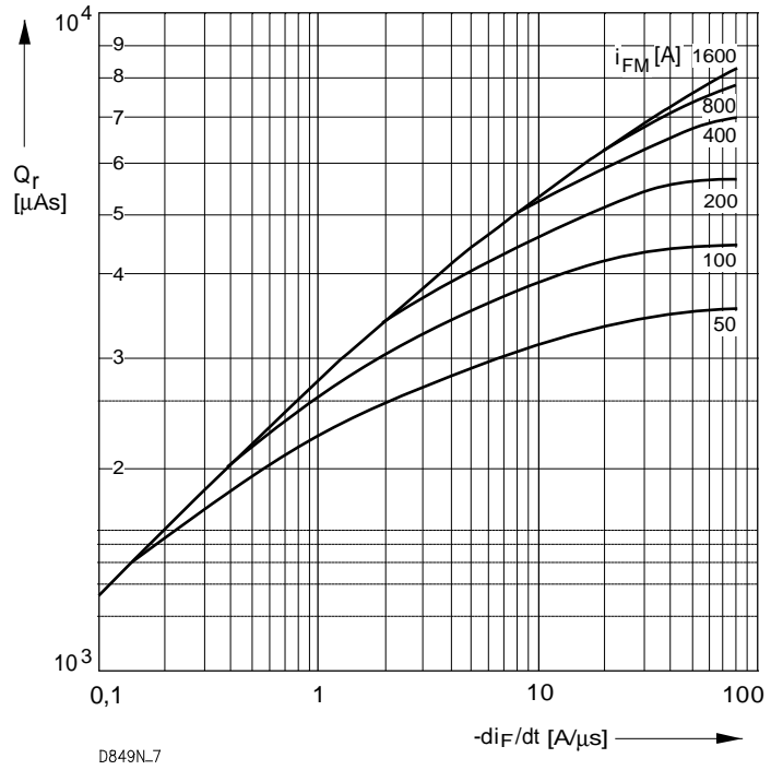
Bild / Fig. 6 Sperrverzögerungsladung / Recovered charge Q_r = \int -di/dt t_{vj} = t_{vjmax} ; v_R \leq 0,5 V_{RRM} ; V_{RM} = 0,8 V_{RRM} Beschaltung / Snubber: C = 1 \mu F ; R = 3,9 \Omega Parameter: Durchlaßstrom / Forward current i_{FM}
